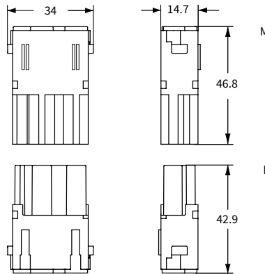
嵌合側 (前面) c ▲マーク側
