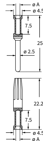
CCF および CCM コンタクト
