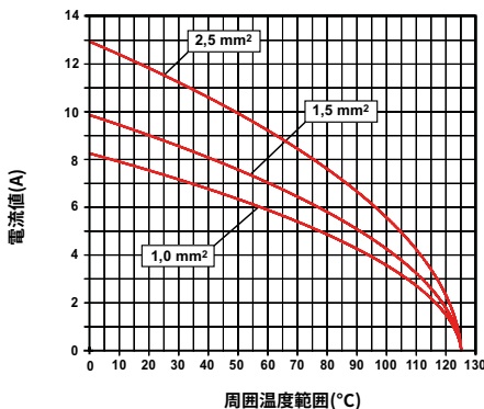
CX 42 D 極 インサート ディレーティング曲線
