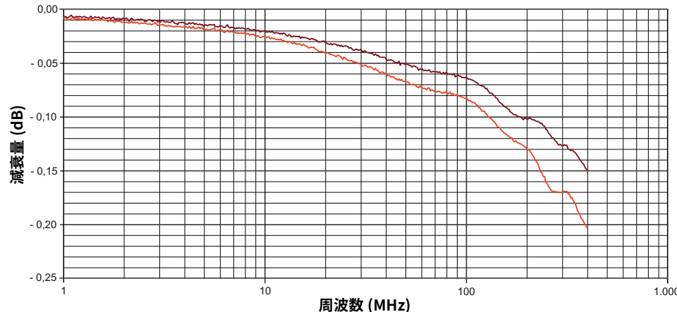
減衰量 (挿入 loss) 75 \Omega 同軸コネクタ (CX 01 BF / BM)
