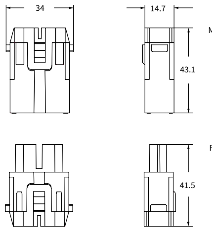
嵌合側 (前面)
