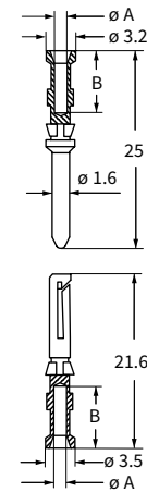
RDF2D および RDM2D コンタクト
