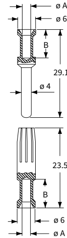
RXF2D および RXM2D コンタクト
