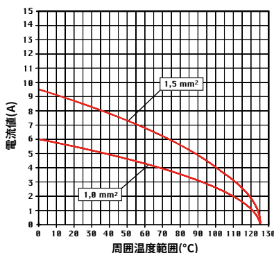
CX 17 極 インサート デレーティング曲線
