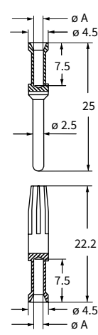
RCF2D および RCM2D コンタクト
