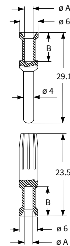
CXF および CXM コンタクト
